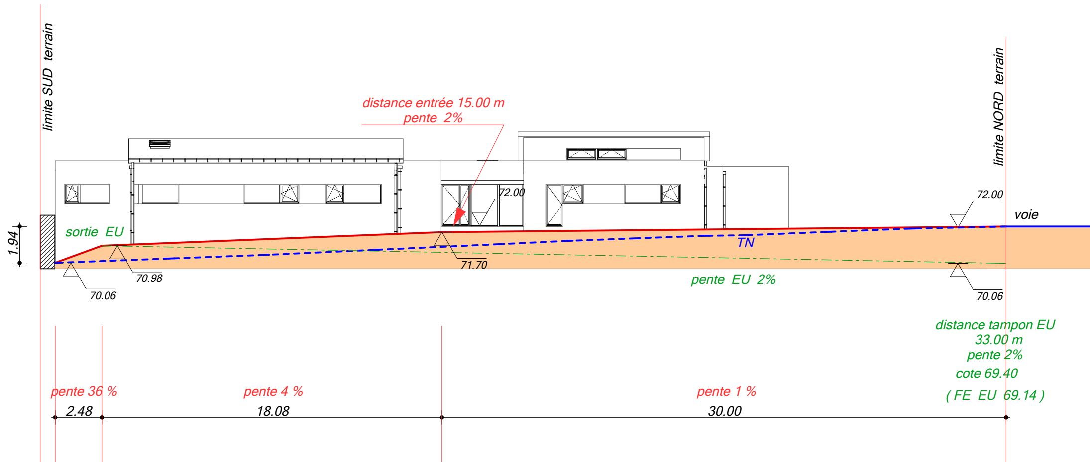
COUPE SUD - NORD ECH 1 / 200 23 mars 2018
