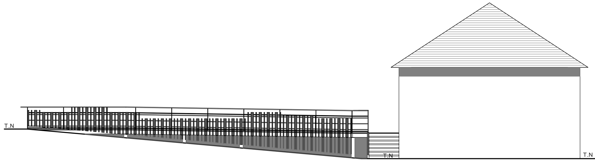
Elévation EST - Echelle 1/100
