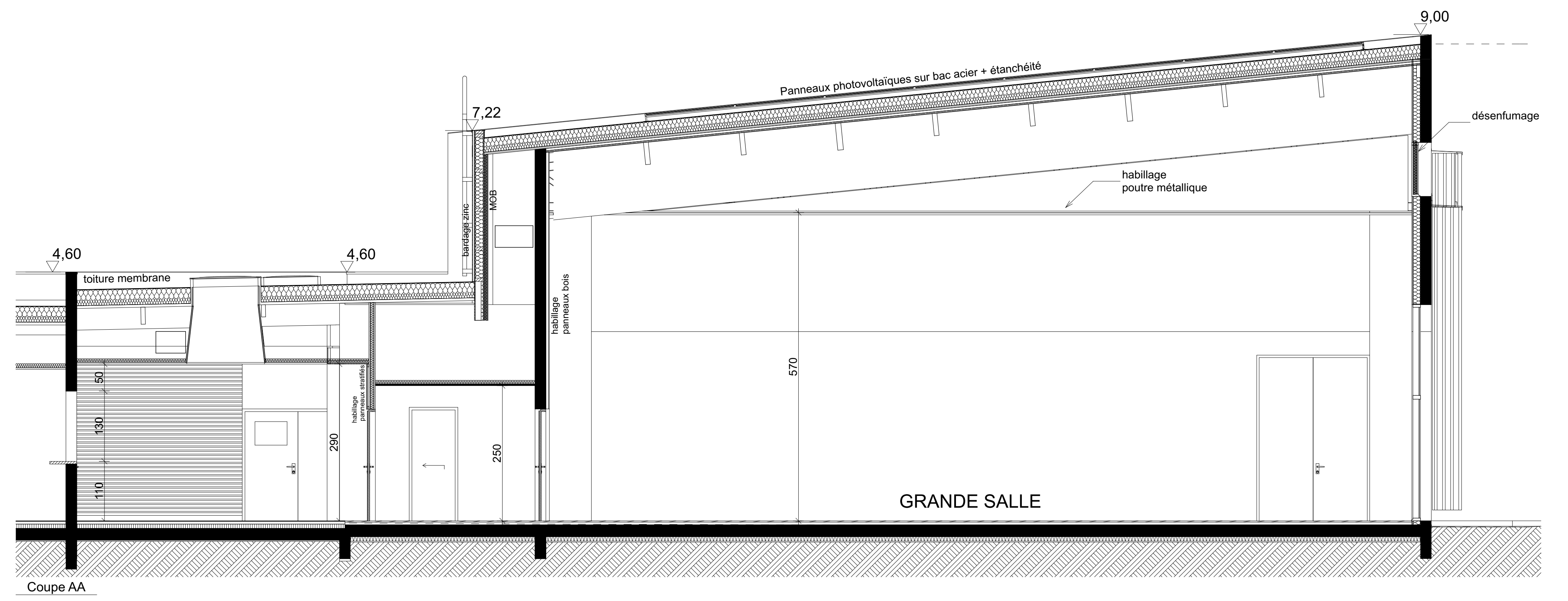
Coupe AA
