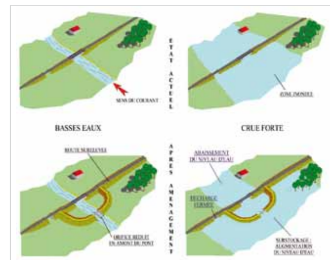
Principe de fonctionnement d'un ralentisseur dynamique (ou bassin).
