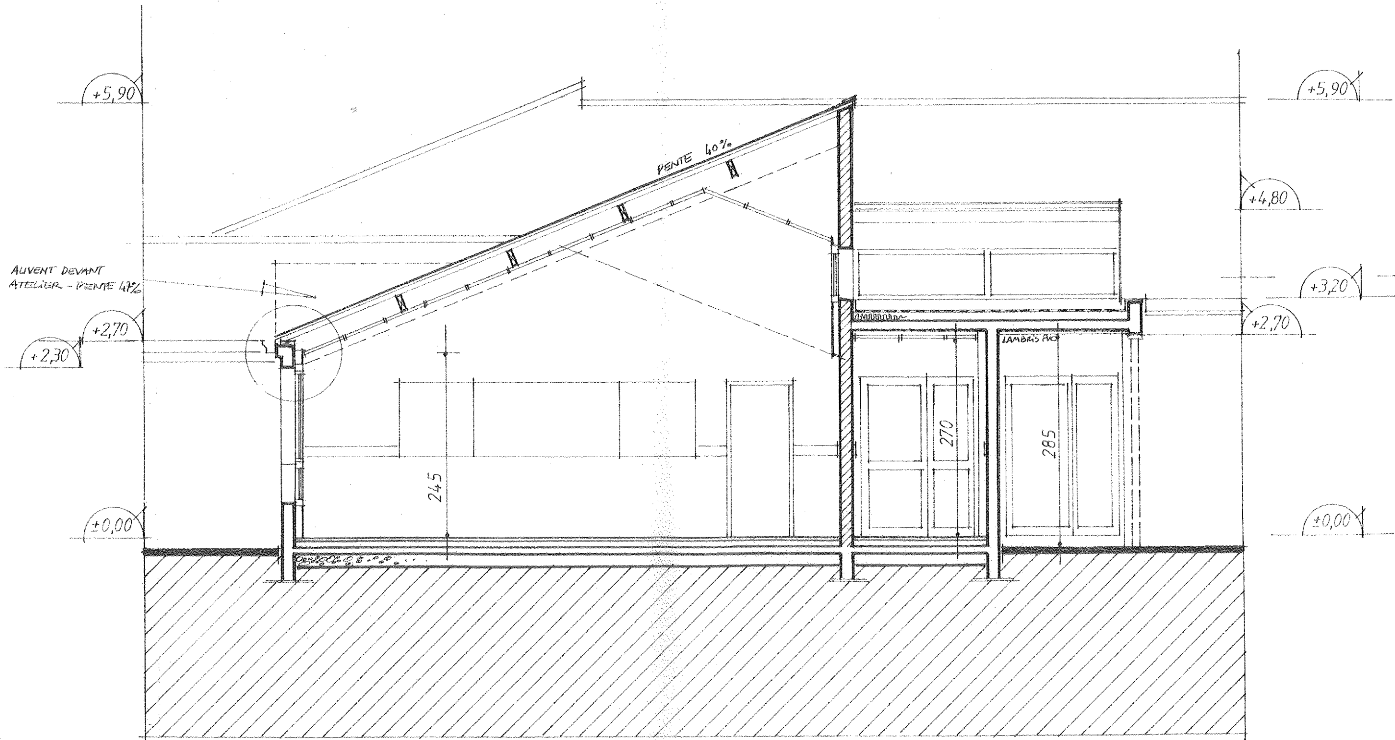
COUPE AA
