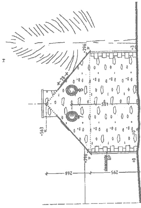
Façade Sud Ouest
