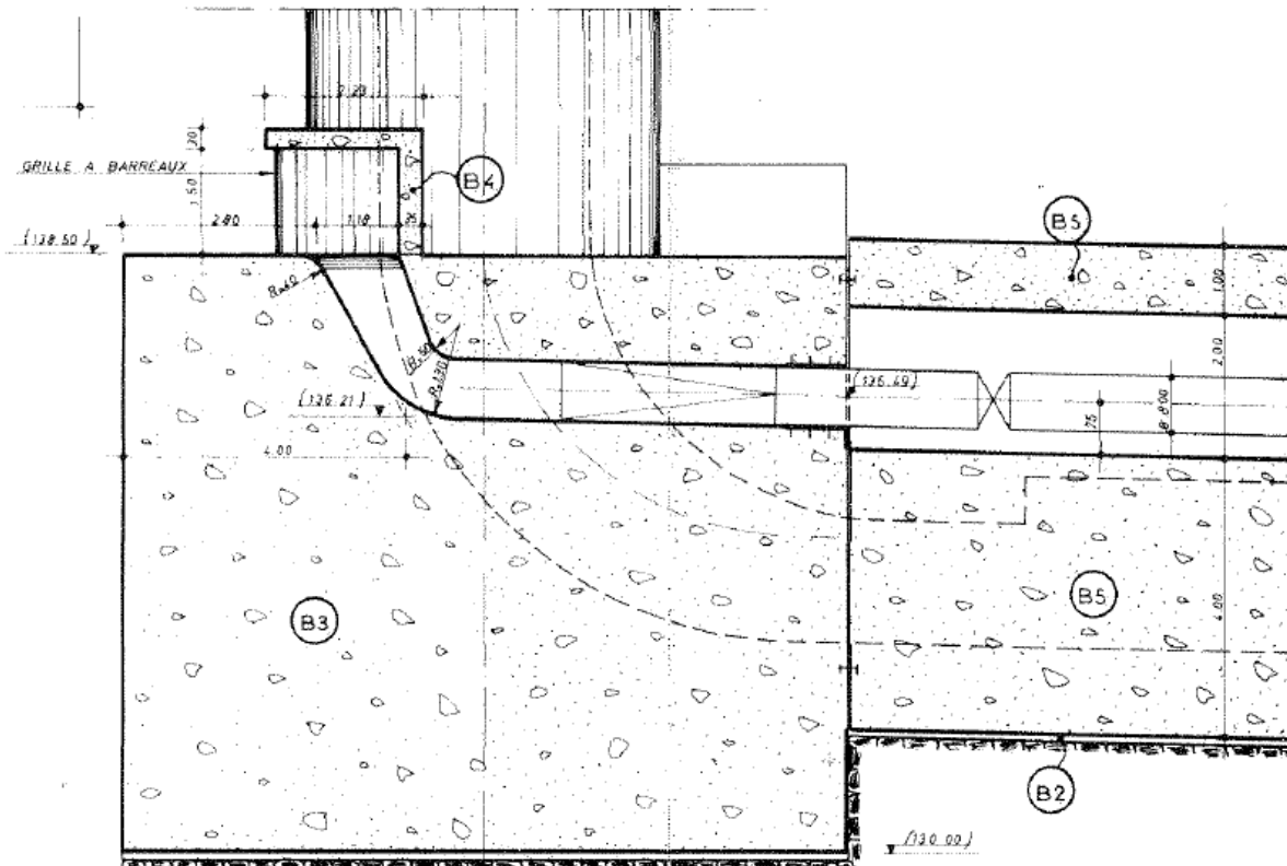
Coupe de l'embranchement de départ de la conduite forcée
