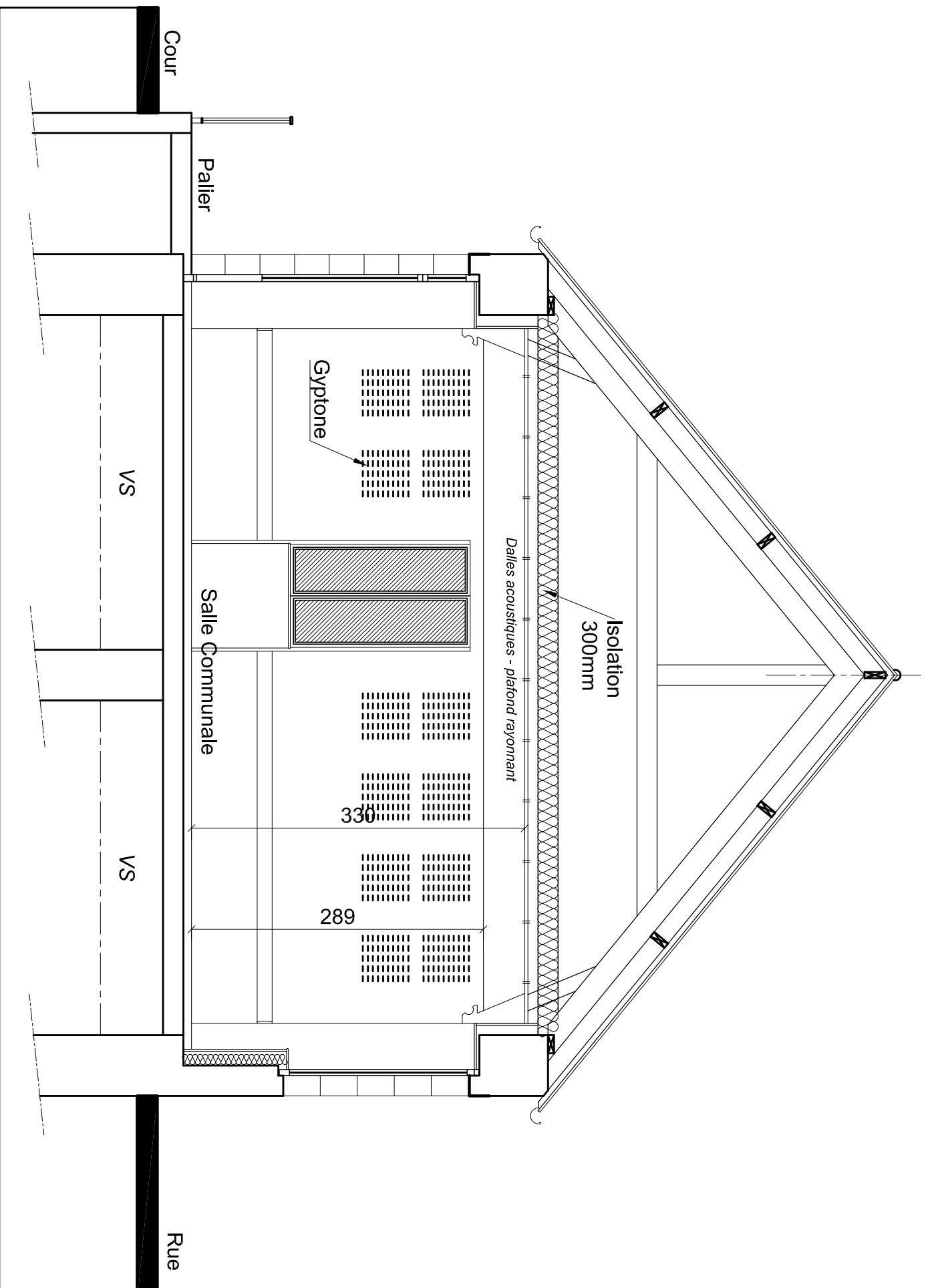
Coupe BB
